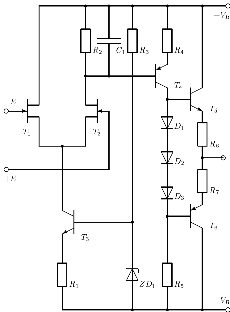
FIGURE 11: Premier essai de symboles électroniques avec \text{\LaTeX}
